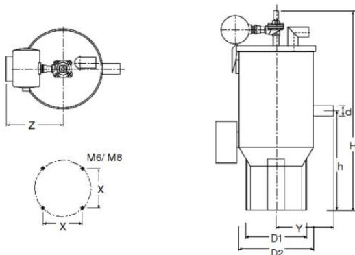
Vacuümhoppers: FX 3534-54 & FX 5134-54
