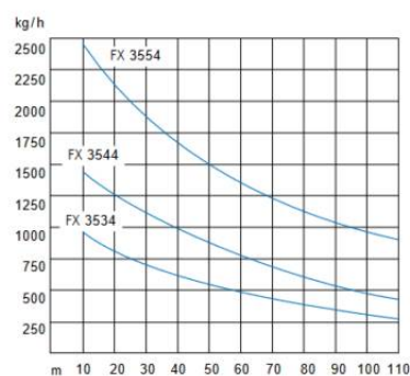
FX-serie 3500 capaciteits diagrammen
