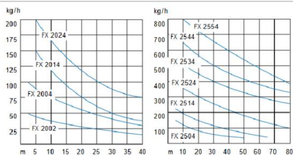
Capaciteits diagrammen Vacuuhoppers - FX-serie
